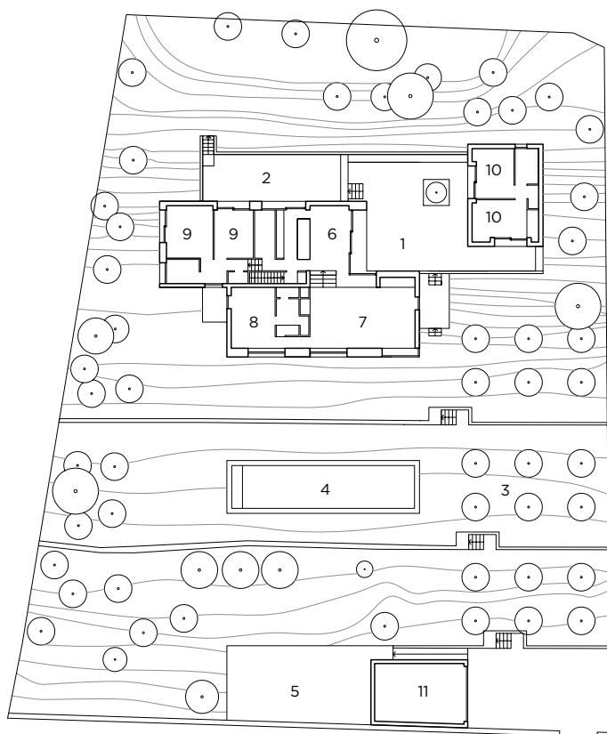
Plan de rez-de-chaussée
